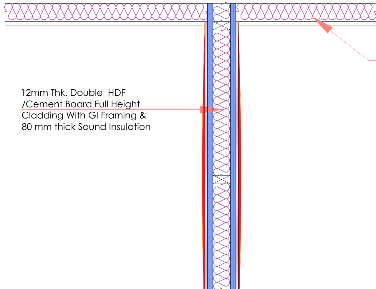
SECTION-A
